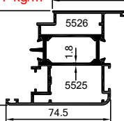
64-5525-5526 2.194 kg/m
