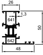
641-642 1.027 kg/m
