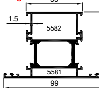
64-4300-4301 2.095 kg/m
