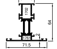
64-1706-1718 1.931 kg/m
