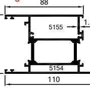
64-4300-4302 2.217 kg/m
