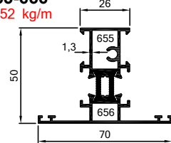
659-660 2.325 kg/m
