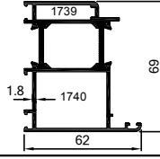
64-1700-1716 1.431 kg/m
